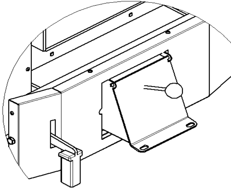
Рисунок 7. Монтаж заслонки
