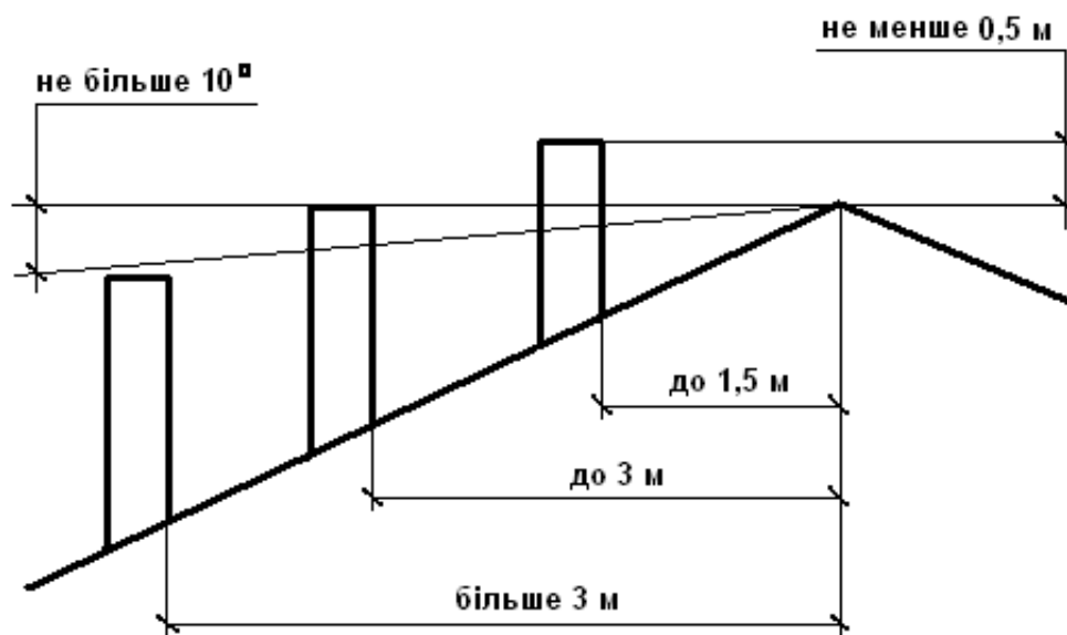
Рисунок 6. Розміщення димоходу
