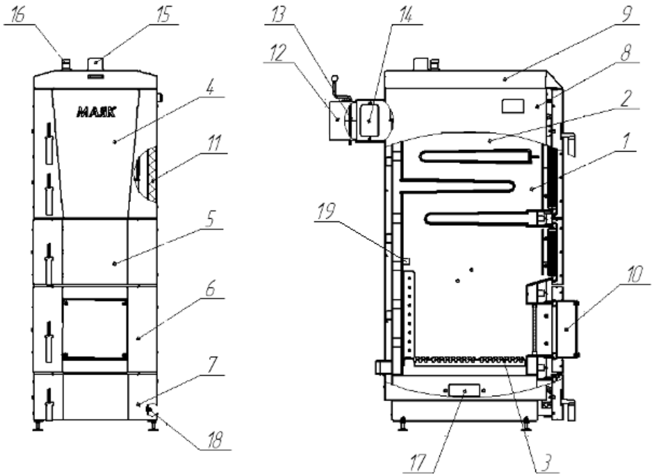
Рисунок 1. Котел опалювальний КТР UNI TYPE H
