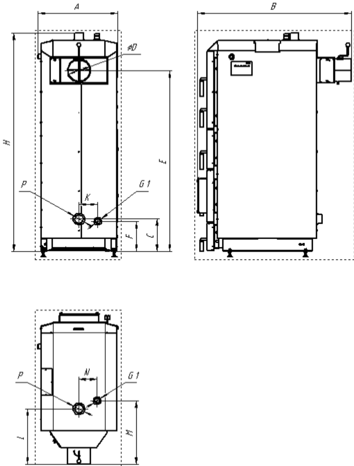
Рисунок 2. Приєднувальні розміри
